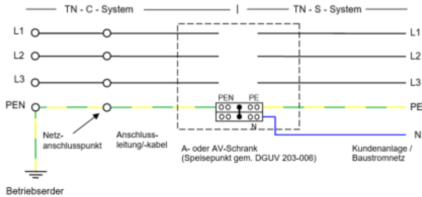
Abbildung 7 - Anschlussmöglichkeiten am Beispiel des TN-C-Systems
