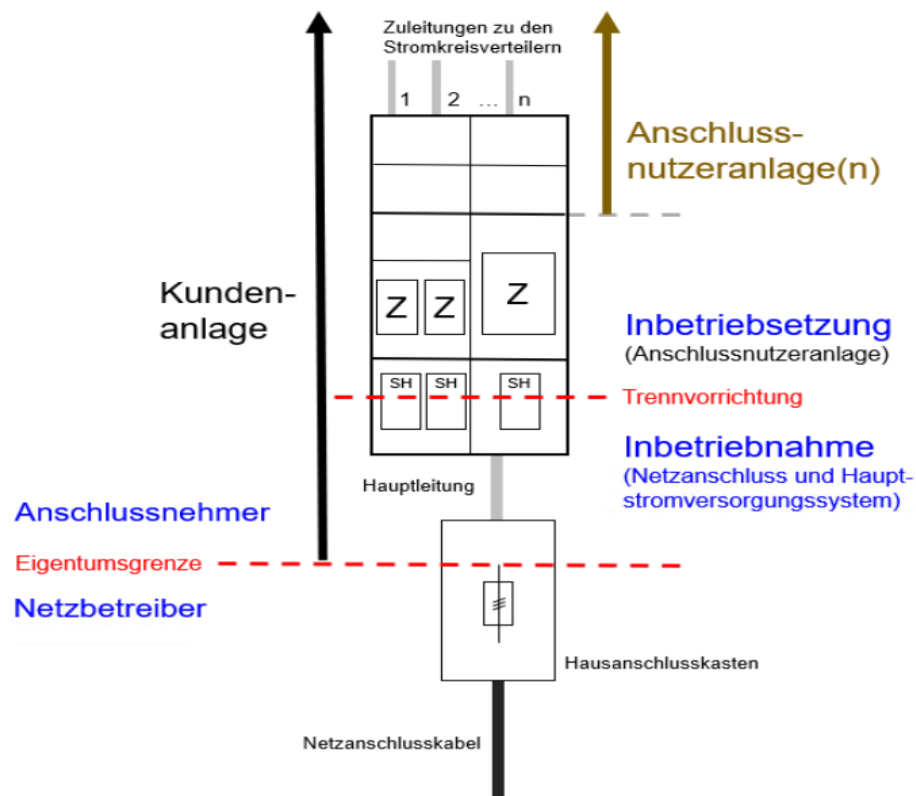
Abbildung 1 - schematische Darstellung der Begriffe Inbetriebnahme / Inbetriebsetzung sowie Kundenanlage / Anschlussnutzeranlage
