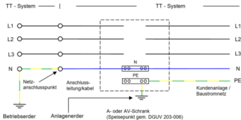
Abbildung 8 - Anschlussmöglichkeiten am Beispiel des TT-Systems
