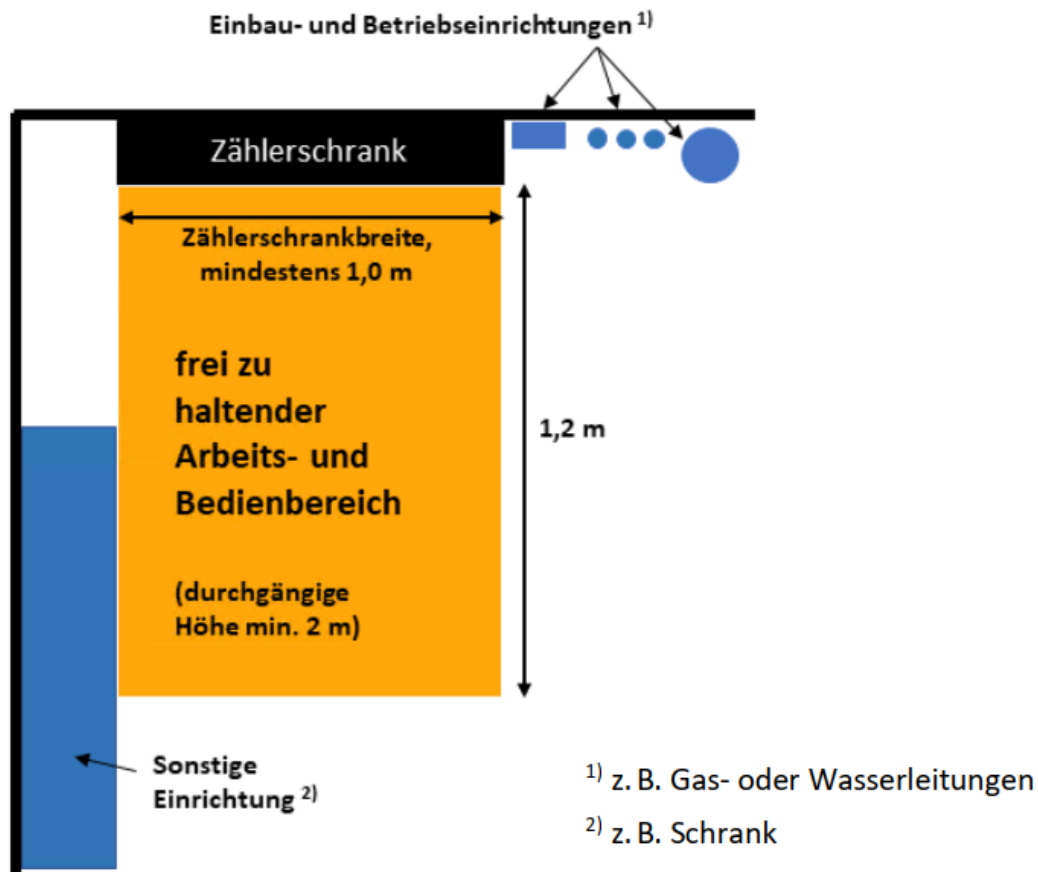
Abbildung 3 - Arbeits- und Bedienbereich vor dem Zählerschrank
